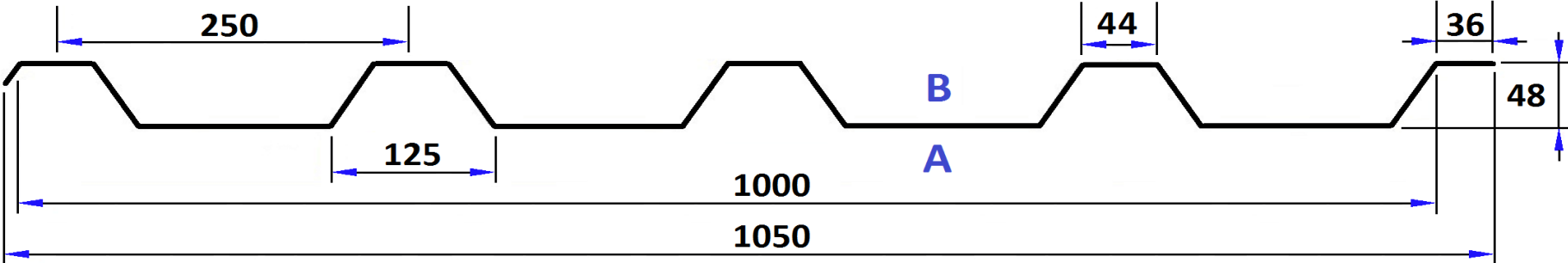
BDC Trapezprofil 50.250 - WAND (Positivlage)
