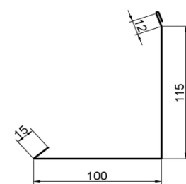
21. Wandanschluss seitlich
