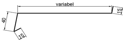
32. Fensterbank
