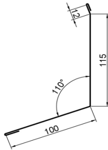
10. Wandanschluss Aufblech 25
