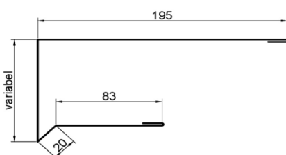
7. Ortgang SW oben U
