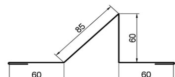
26. Schneestopper mitte
