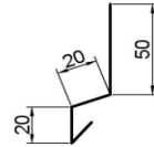
30. Tropfkante Form B
