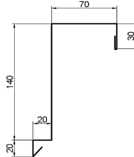
17. Ortgang Paneeldach 30
