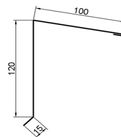
6. Pultabschluss 25
