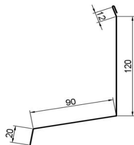
20. Wandanschluss Aufblech seitlich
