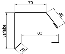
16. Ortgang SW seitlich U
