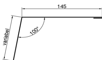
24. Traufenblech SW
