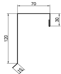
18. Ortgang Paneeldach 25
