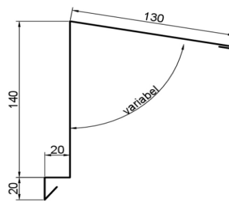
5. Pultabschluss 33
