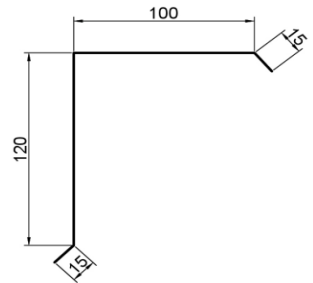
14. Ortgang Aufblech 25 seitlich
