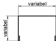
35. U Abdeckprofil
