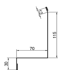
19. Wandanschluss Paneeldach seitlich 25
