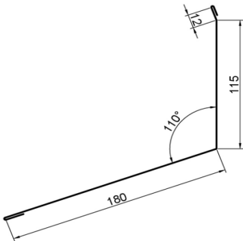
9. Wandanschluss Aufblech 33
