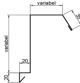
13. Ortgang Aufblech V seitlich
