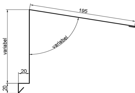
4. Ortgang SW oben L
