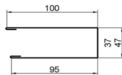
8. Pultabschluss U für Trapez
